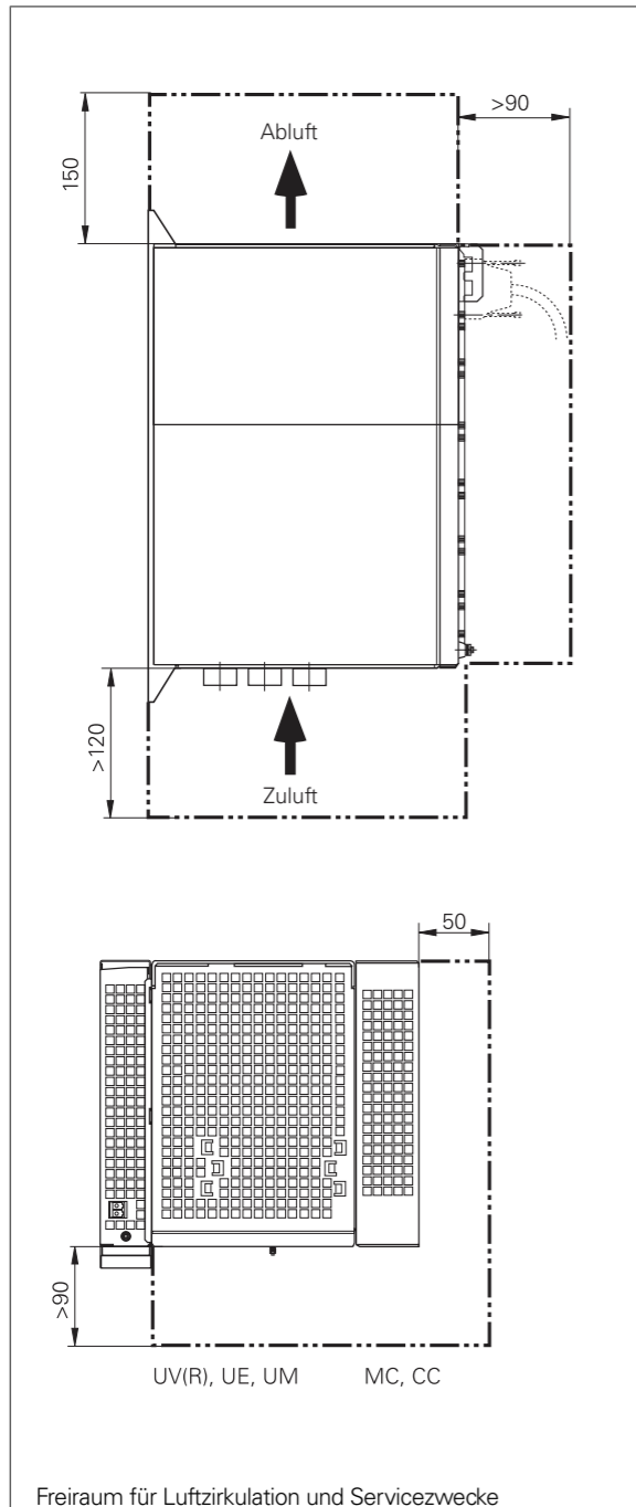
Einbau in Schaltschrank
