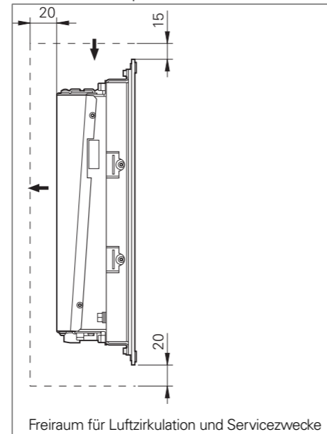
Einbau in Bedienpult
